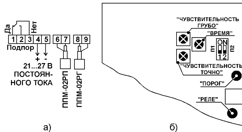
Рис. 8. Схема подключения и органы регулировки датчика РСУ-1РА.
