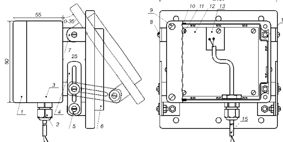
Рис. 5. Конструкция генератора ППМ-02РГ и детектора ППМ-02РП.
