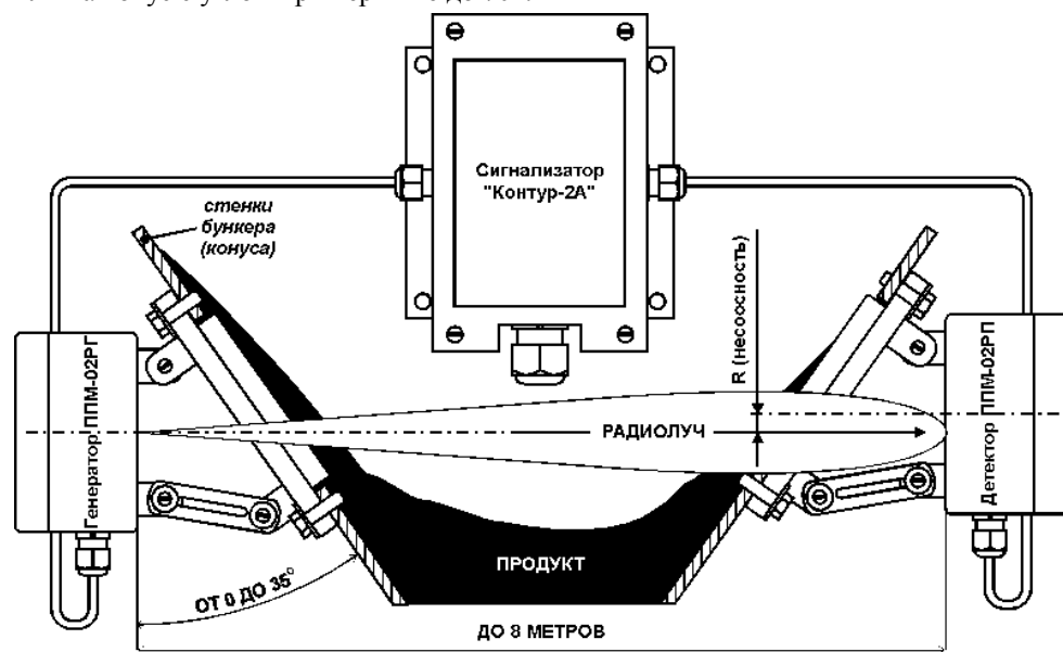
Рис. 1. Принцип действия датчика РСУ-1РА.
