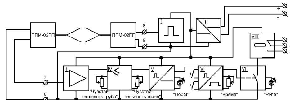
Рис. 2. Структурная схема датчика РСУ-1РА.
